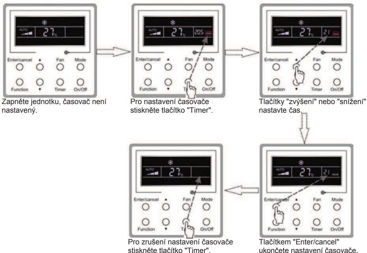
Obr. 8: Nastavení časovače na vypnutí v "zapnutém" stavu jednotky
